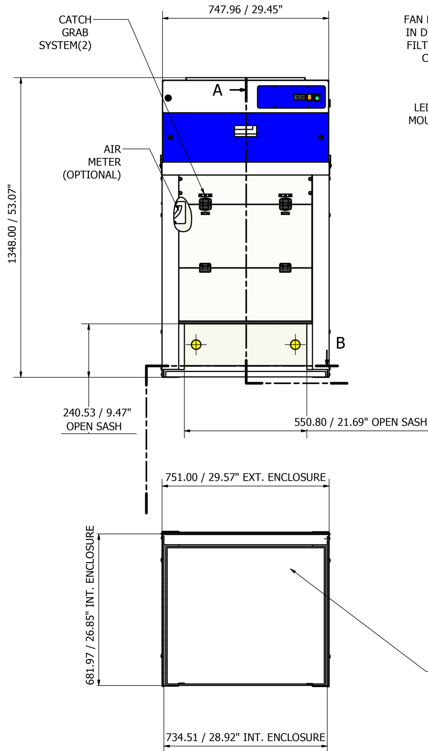
B-B ( 1 : 10 )
