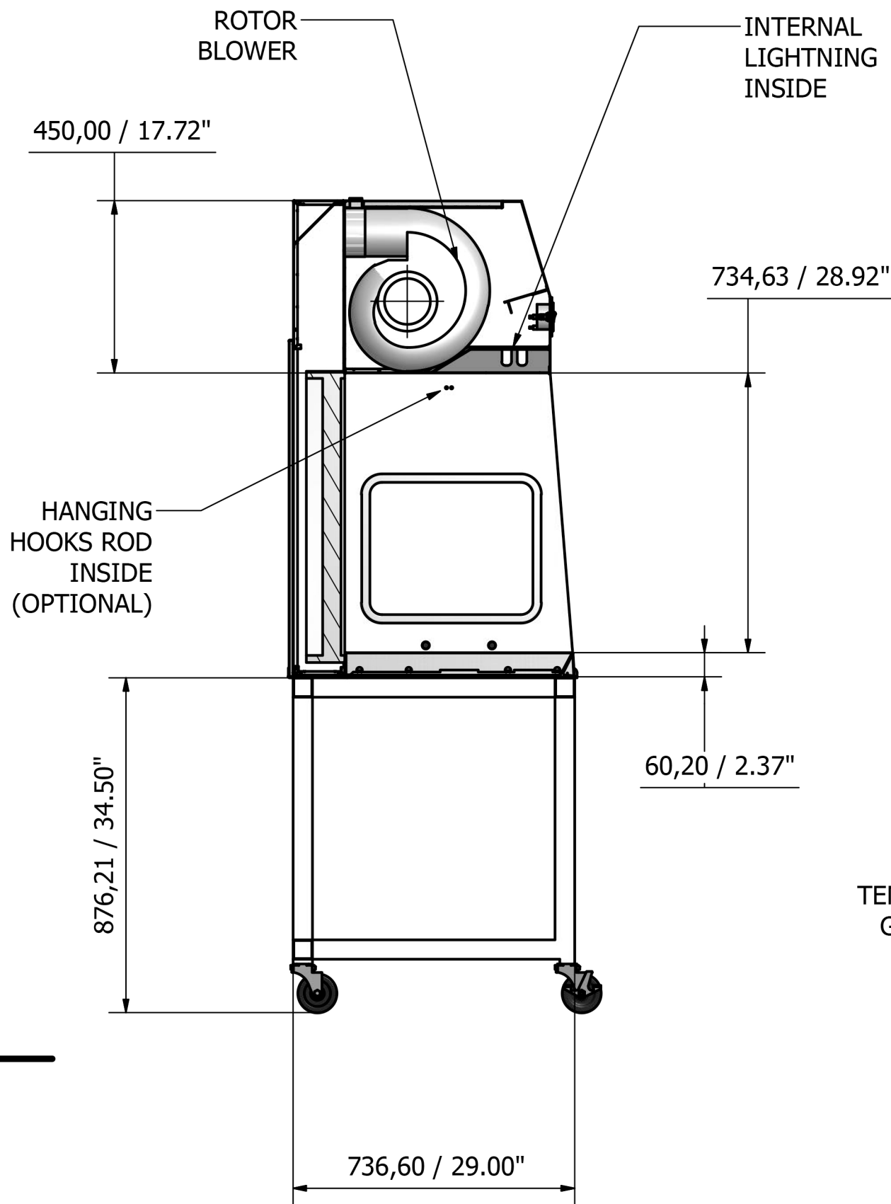
A-A ( 1 : 14 )
