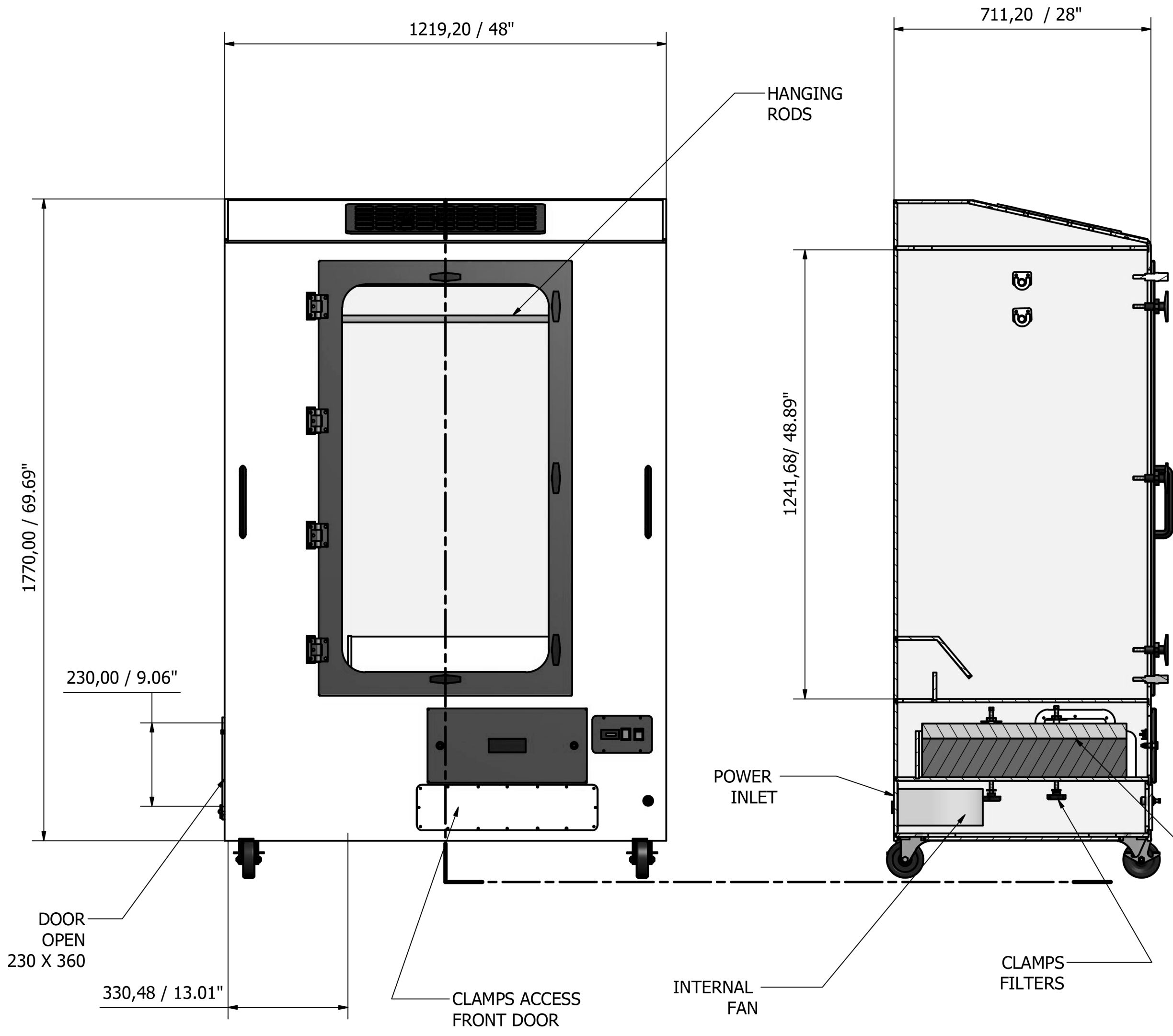
A-A ( 1 : 10 )
