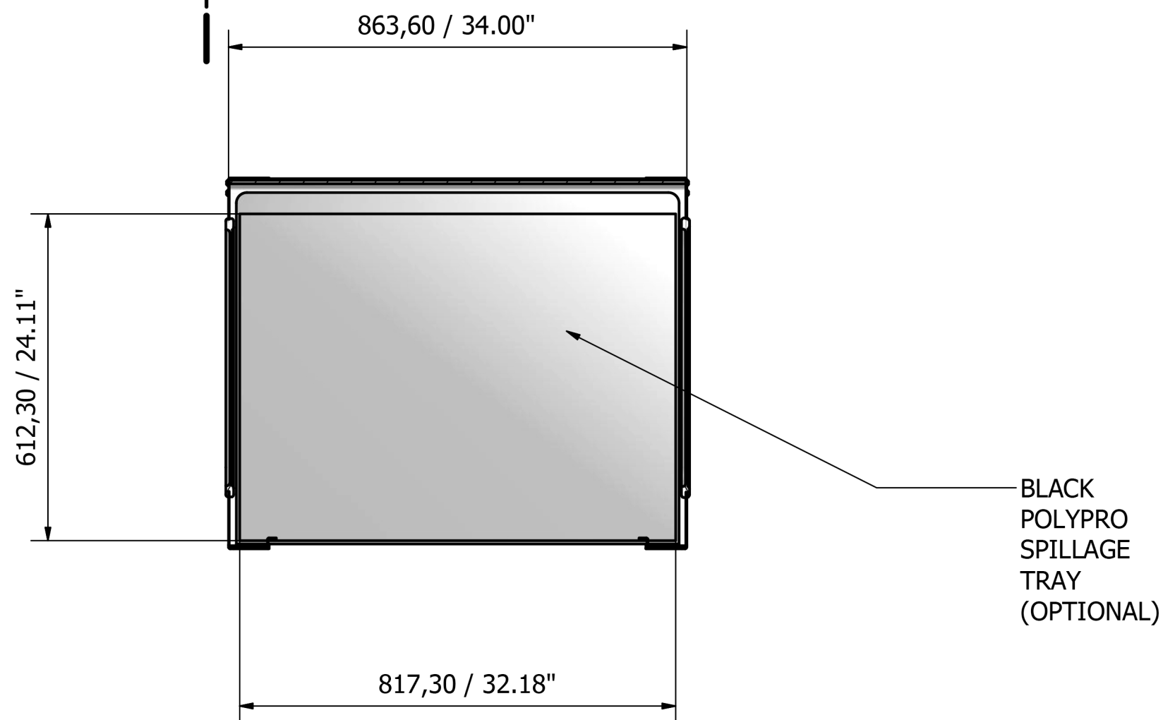
A-A ( 1 : 10 )
