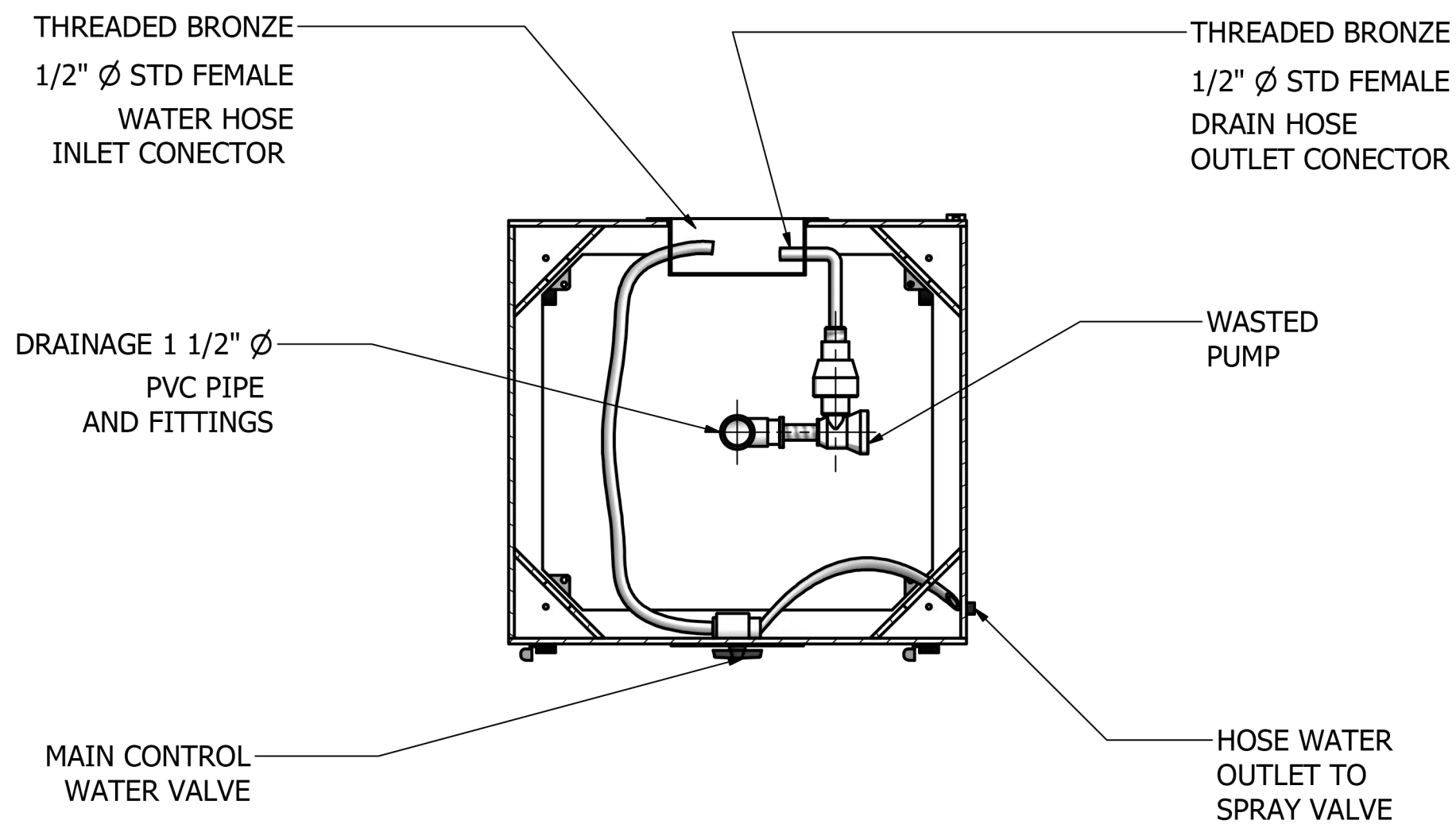
B-B ( 1 : 10 )
