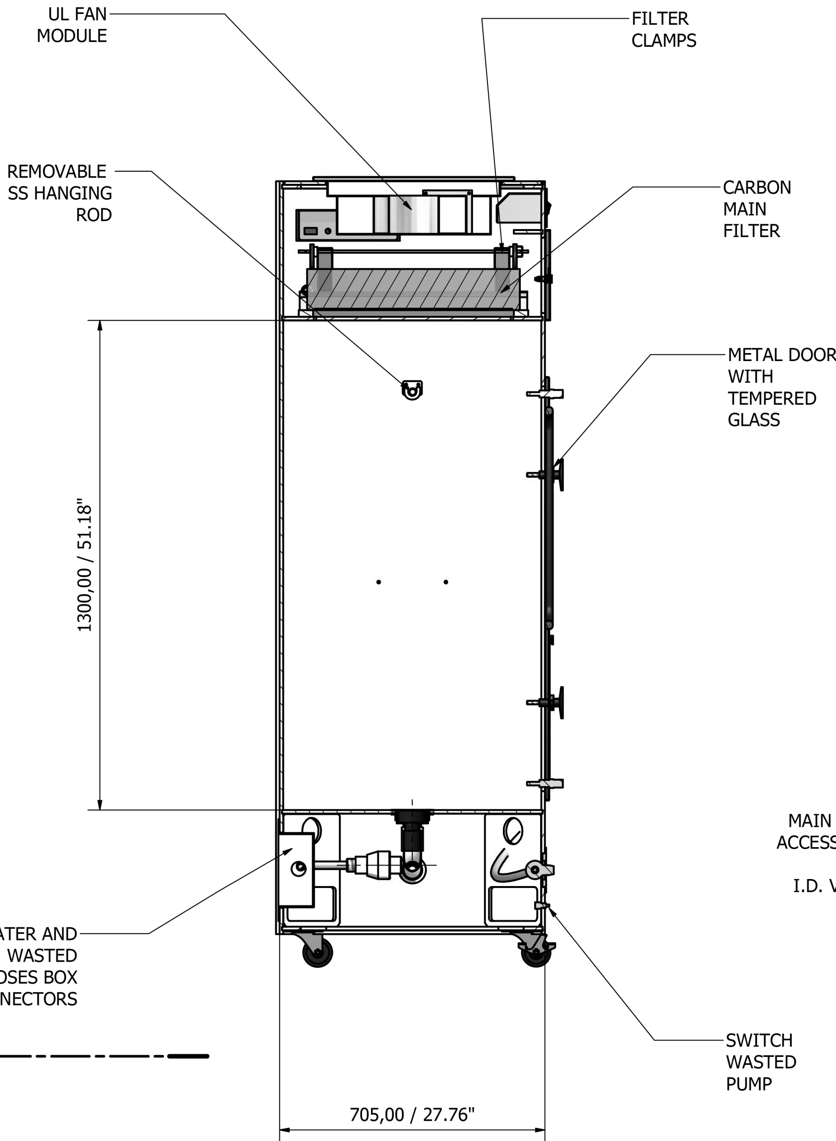
A-A ( 1 : 10 )
