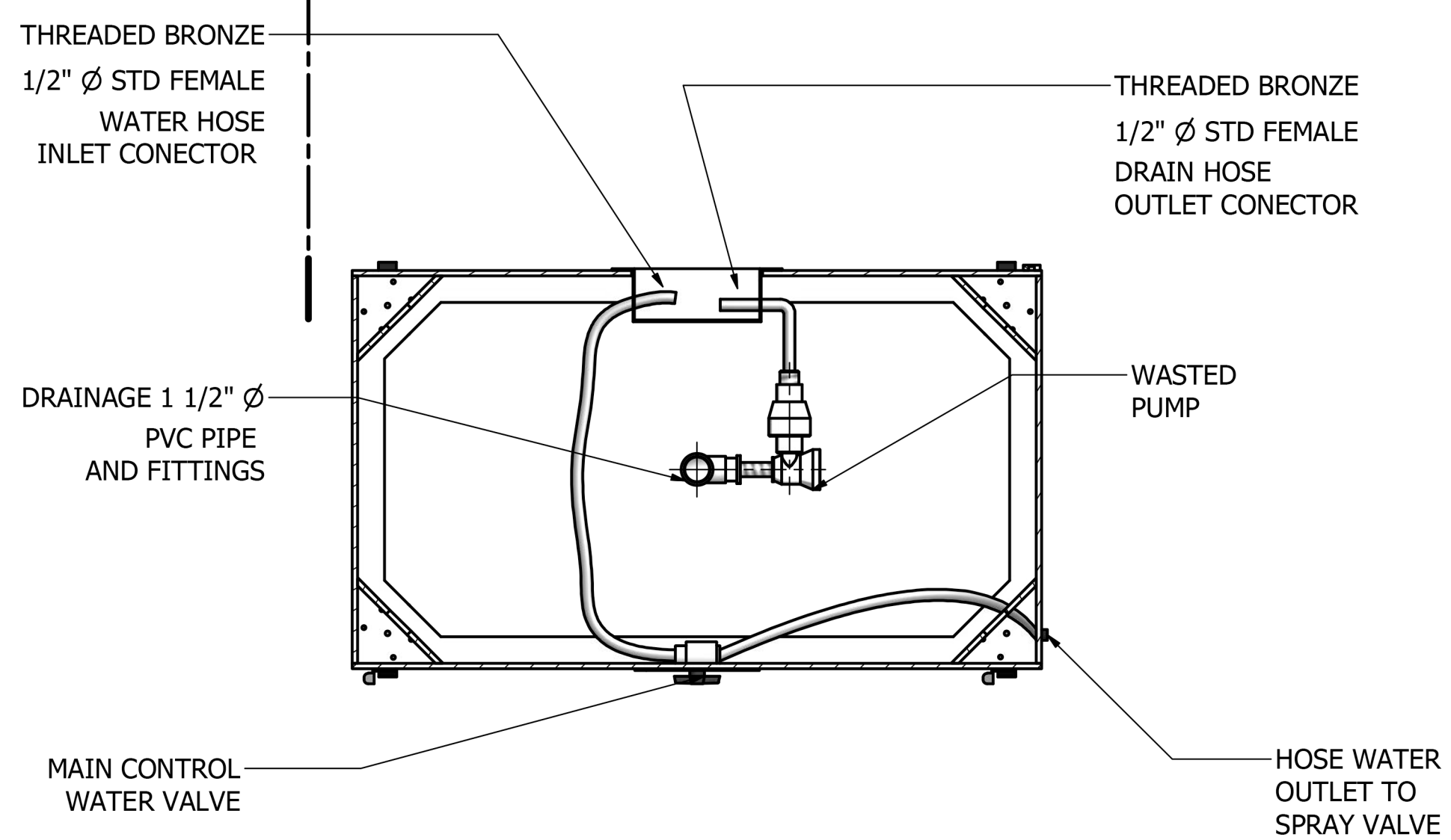
B-B ( 1 : 10 )
