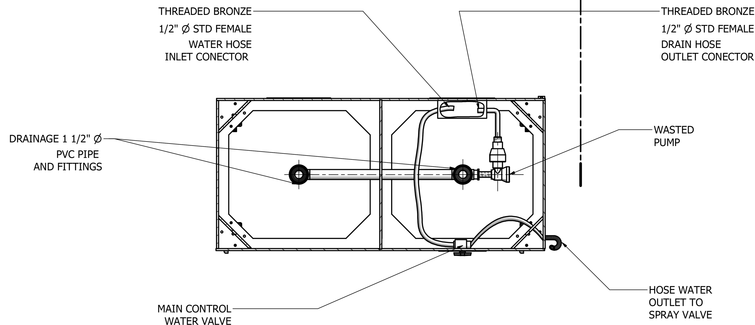
B-B ( 1:10 )
