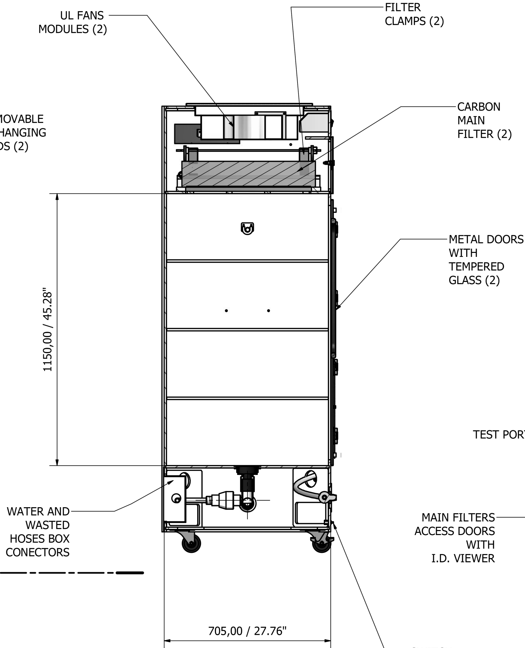
A-A ( 1:10 )
