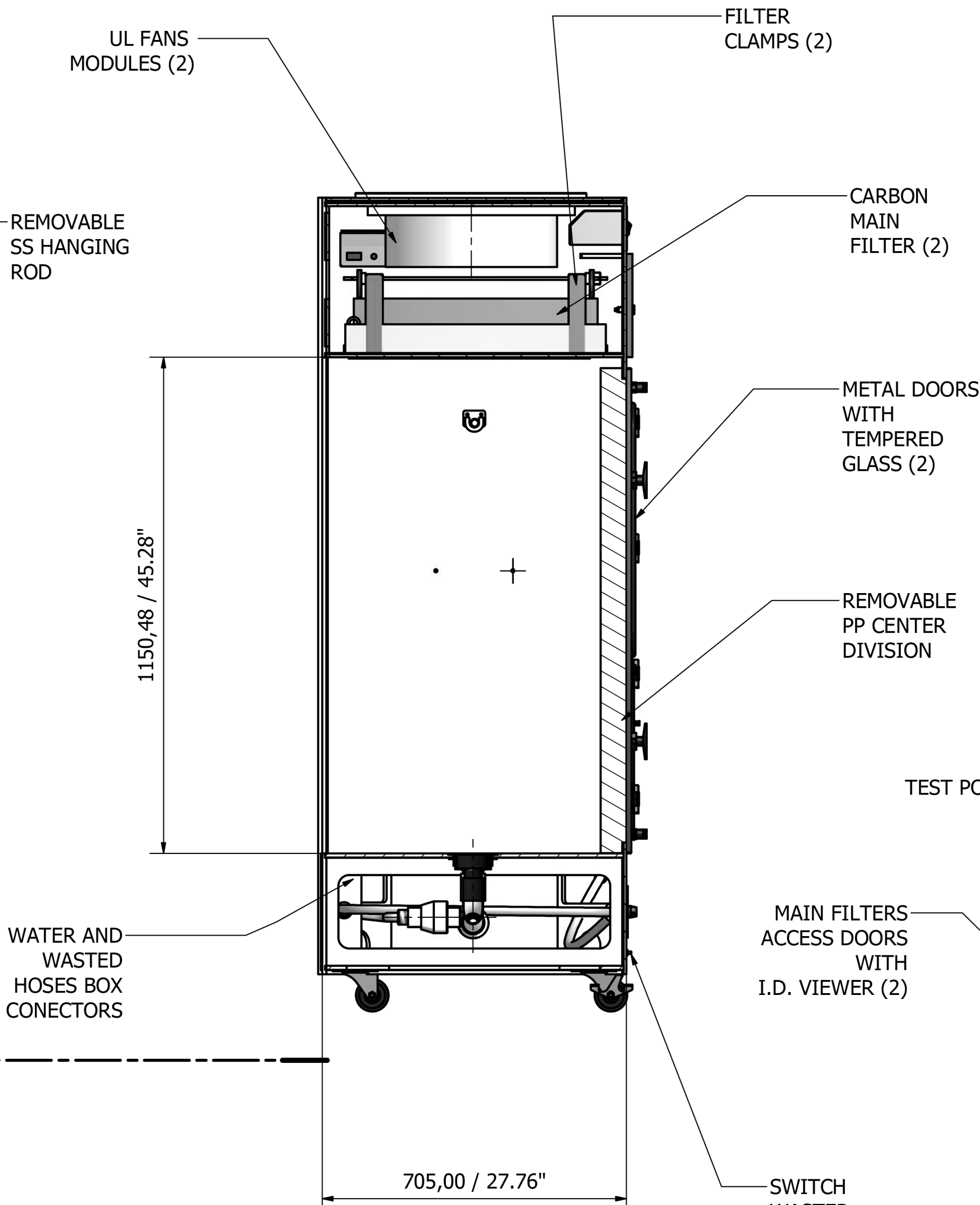
A-A ( 1 : 10 )
