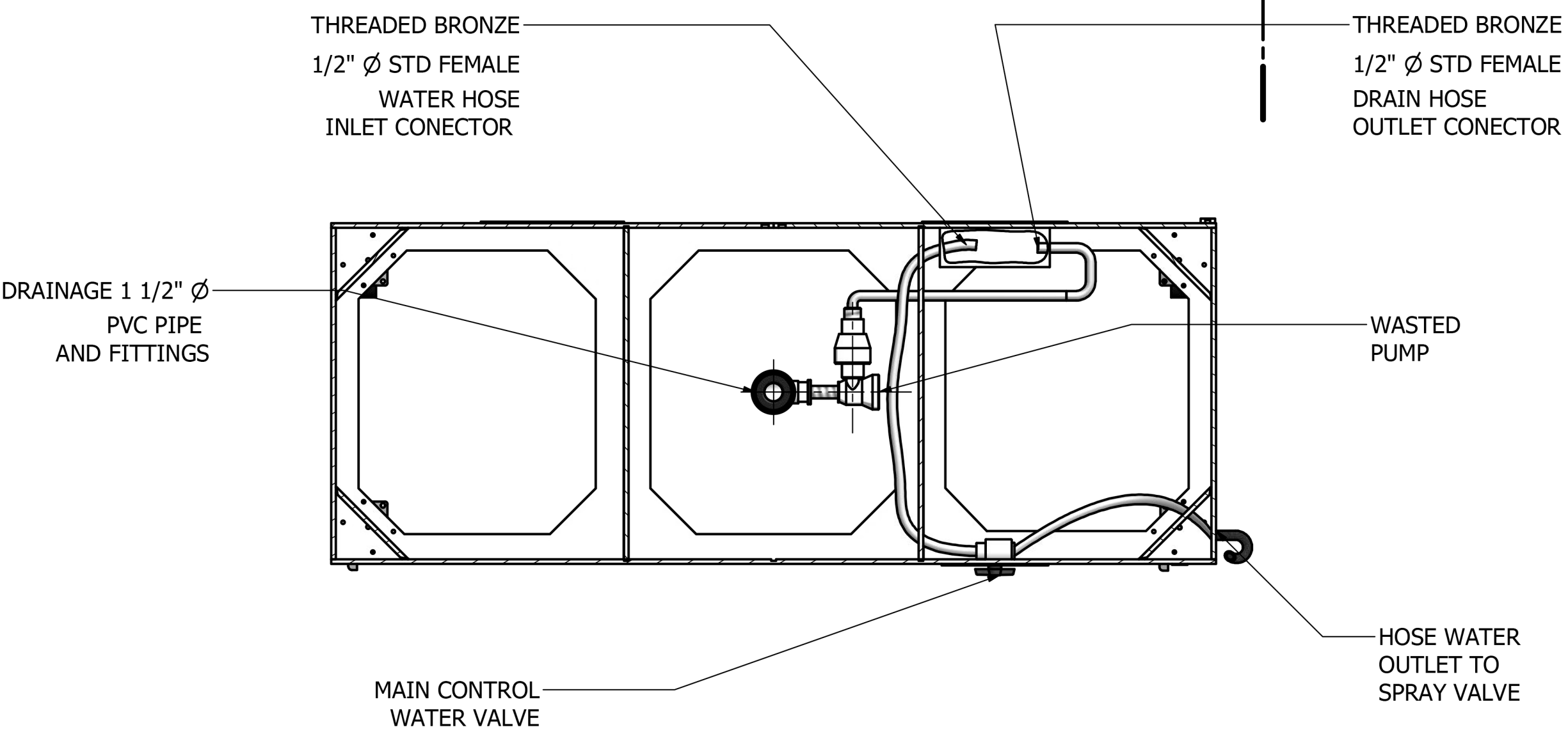
B-B ( 1 : 10 )
