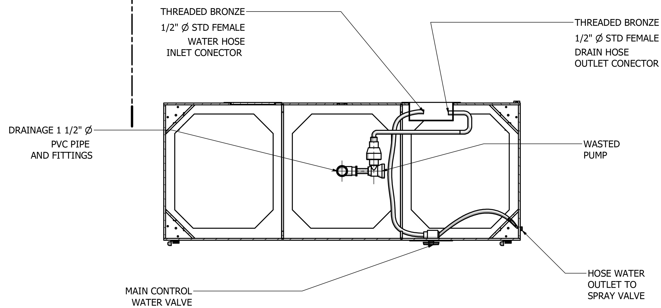
B-B ( 1 : 10 )
