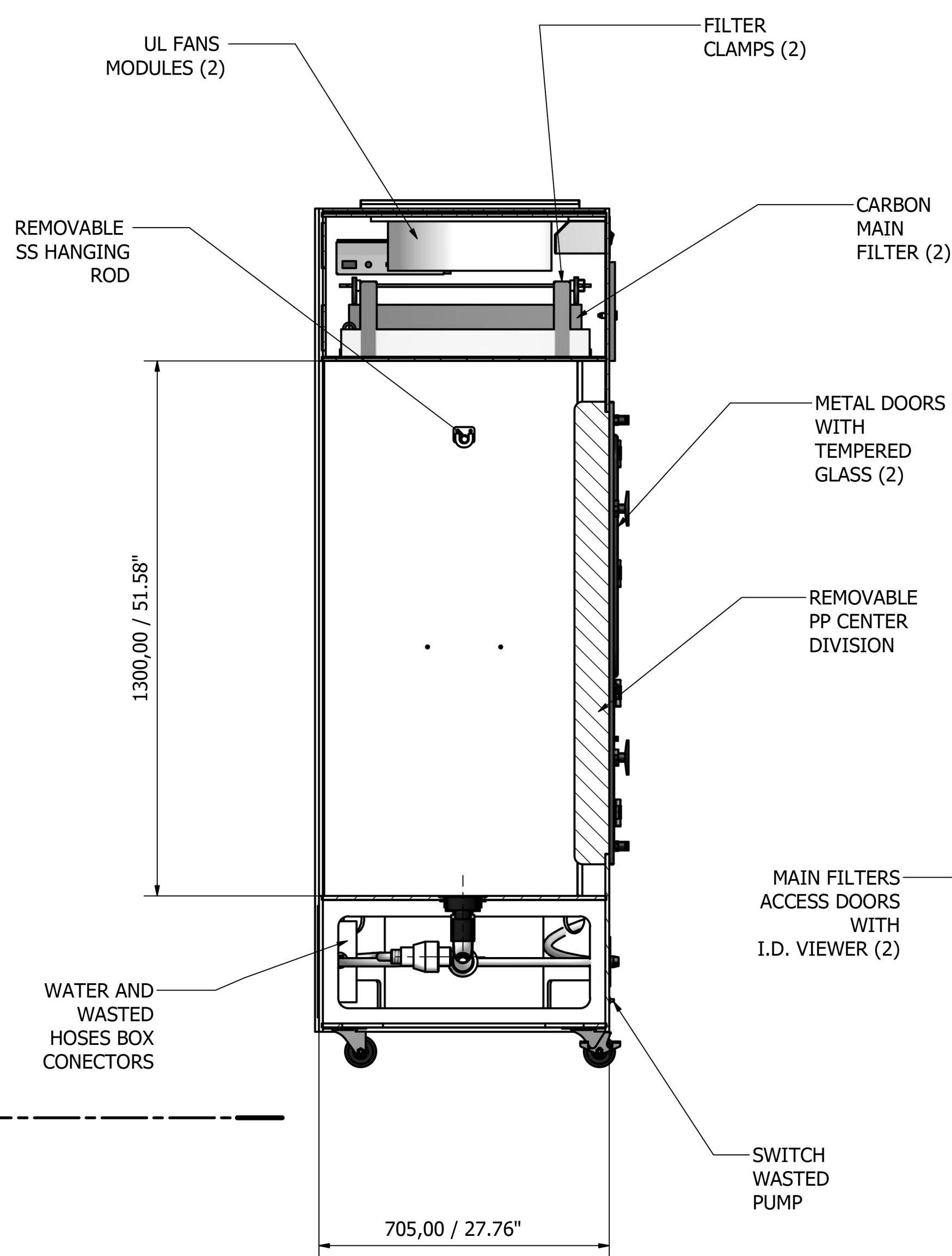
A-A ( 1 : 10 )
