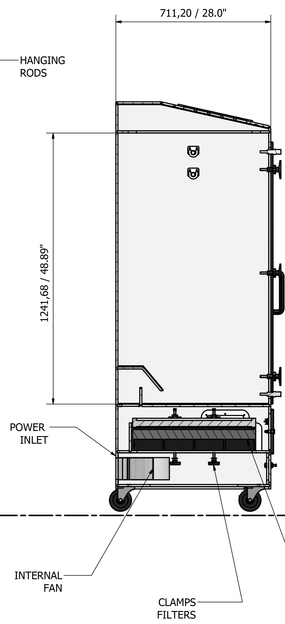
A-A ( 1 : 10 )
