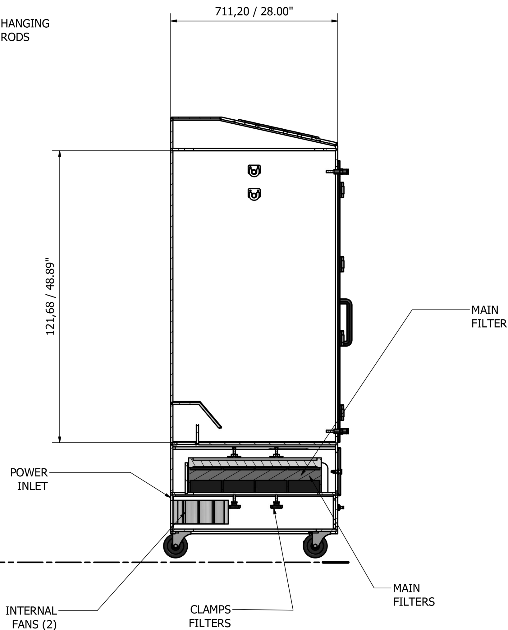
A-A ( 1 : 10 )
