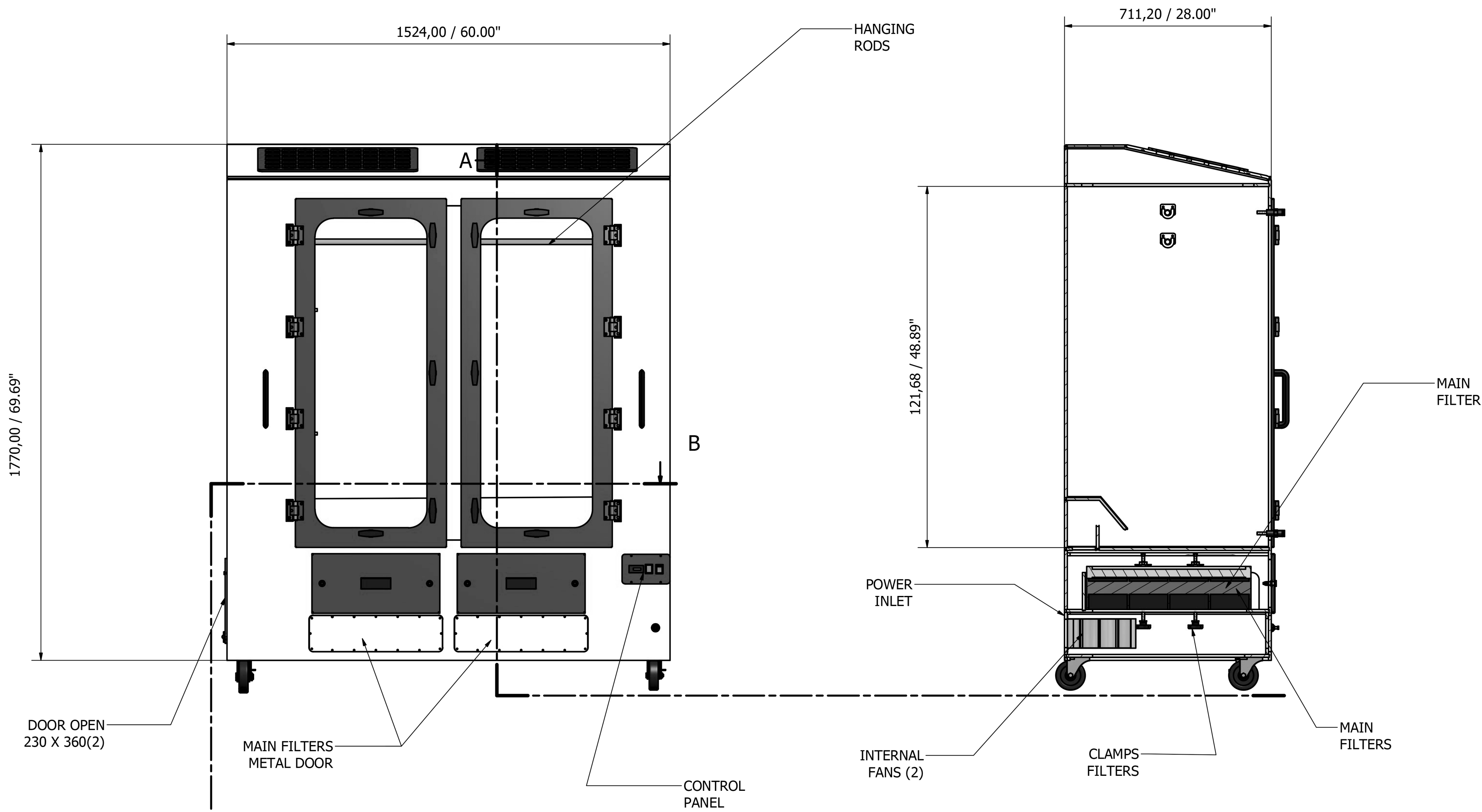
A-A ( 1 : 10 )
